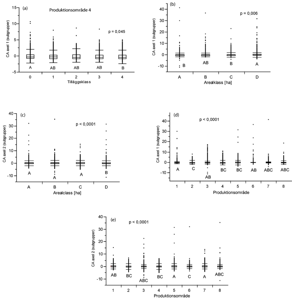
Figur 10: Signifikanta skillnader i position längs CA-axel 1 och 2 mellan (a) tilläggsklasser, (b) & (c) arealklasser och (d) & (e) produktionsområden testat med Tukey's HSD post hoc tester. Nivåer markerade med olika bokstäver skiljer sig signifikanta från varandra.
