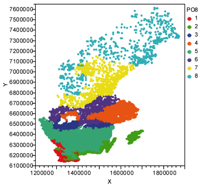
Figur 2: Samtliga TUVAs-objekt, indelade i åtta produktionsområden (PO8).
