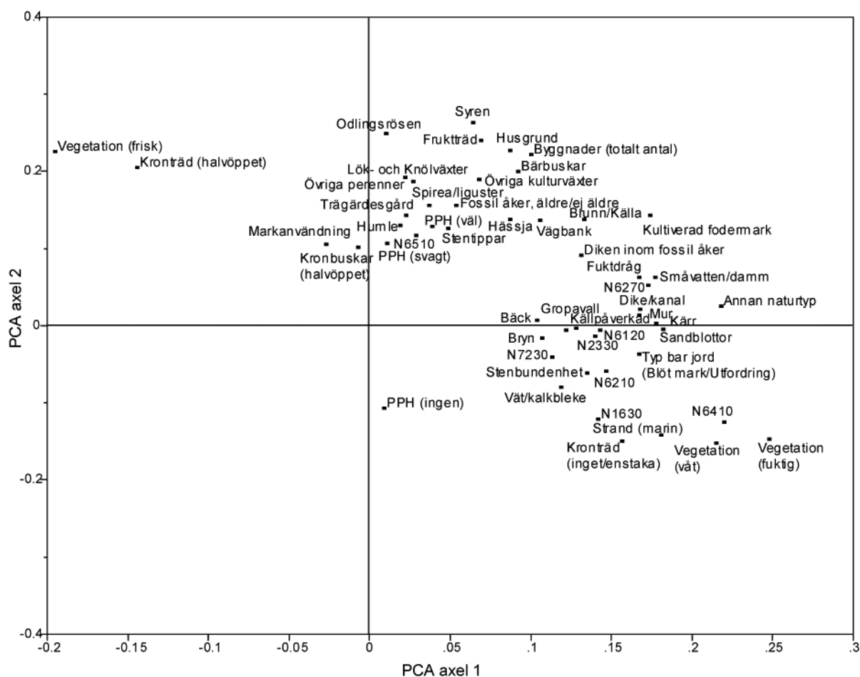
Figur 4: PCA-diagram som visar likheter och skillnader mellan de viktigaste (koordinater > 0,1) oberoende miljövariablerna (n = 52) som ingår i TUVU-databasen. Denna fördelning av miljövariabler ligger till grund för spridningen av objekt i figur 3.
