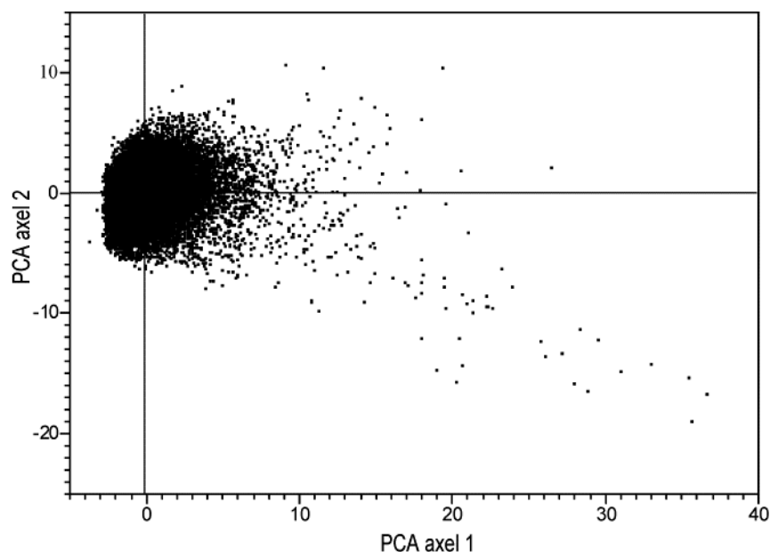
Figur 3: PCA diagram som visar samtliga objekt som ingår i TUVAdatabasen ( n = 47\,467 ), fördelade efter likhet och olikhet i 108 olika variabler som beskriver objekten. Variablerna fördelning presenteras i figur 4. Egenvärden axel 1: 0,034; axel 2: 0,034.
