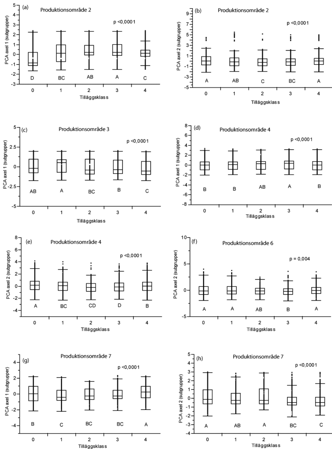
Figur 7: Signifikanta skillnader i TUVA-objektens position längs PCA axel 1 och 2 mellan (a) & (b) tilläggsklasser i produktionsområde 2, (c) i produktionsområde 3, (d) & (e) i produktionsområde 4, (f) i produktionsområde 6, och (g) & (h) i produktionsområde 7 testat med Tukey's HSD post hoc tester. Nivåer markerade med olika bokstäver skiljer sig signifikanta från varandra.
