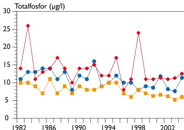
Figur 5. Totalfosforhalt i ytvatten (0,5 m) vid M1 och M2 i Mariestadsfjärdens, samt vid Dagskärsgrund i Storsjön. Samtliga data är medelvärden för resp. provtagningssäsong 1982-2004. Symboler enligt figur 3.
